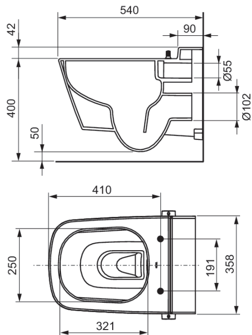
TECEone bidé WC-istuin
