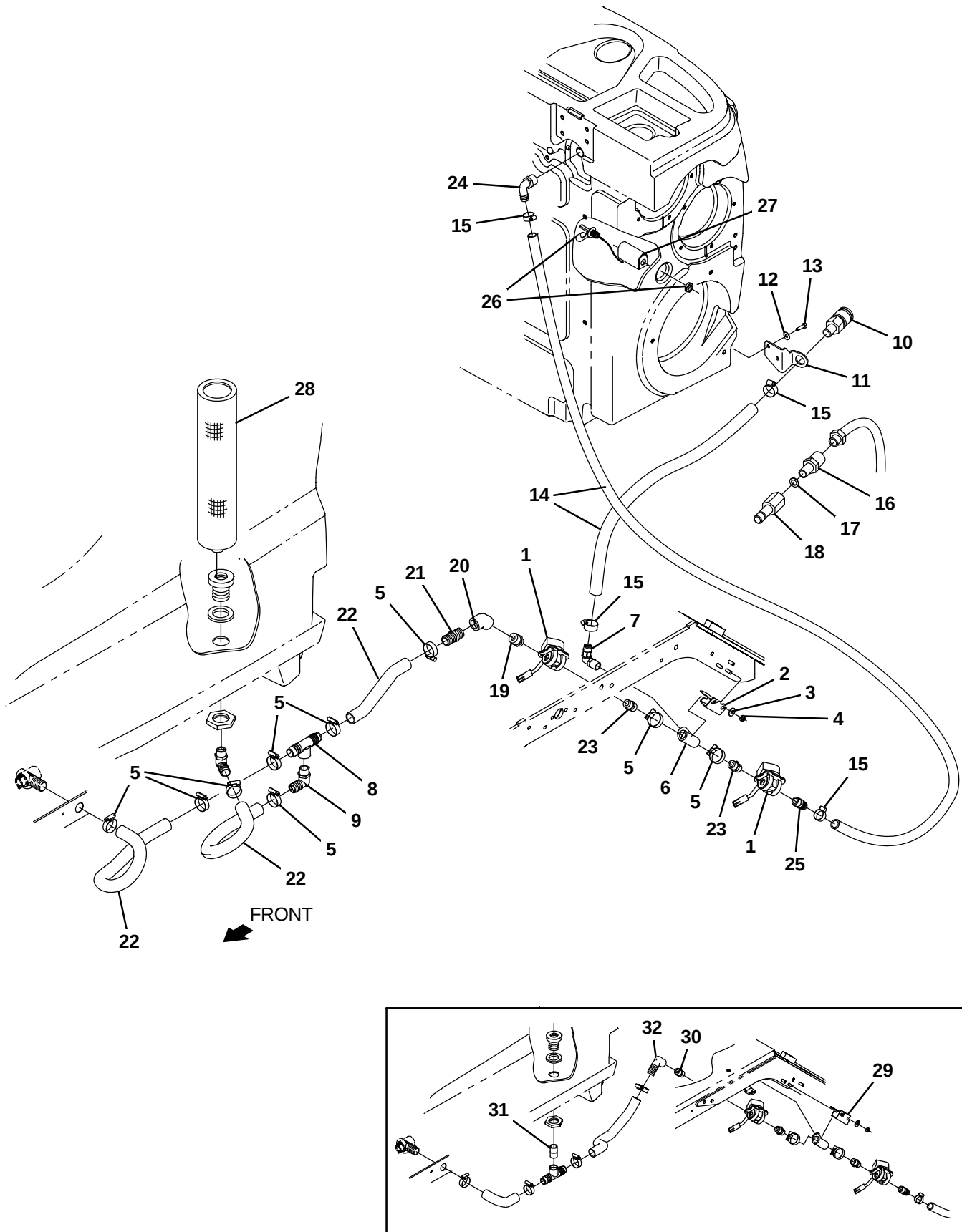
Fig. 28 – ES Auto Fill Group
