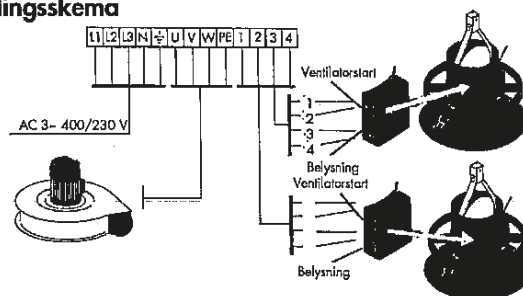
Startapparat SA-24/75-2 koblet til 2 stk. punktudsug (PlymoVent LM-2) med fælles ventilator FS-3000 og belysning i trage på udsugningsarmene.
