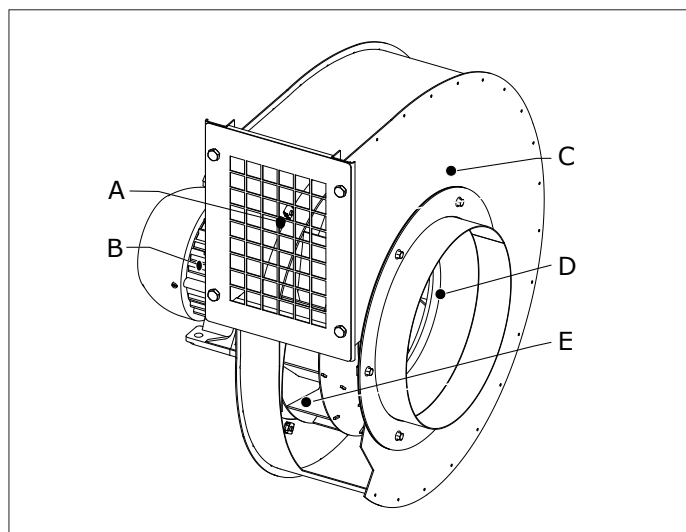
Fig. 2.2 Huvudkomponenter FUA-3000/4700
