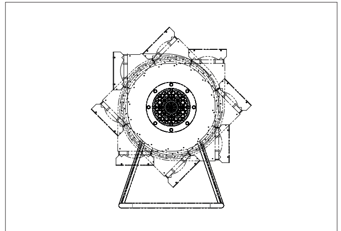
Fig. 4.3 Variable Auslassposition
