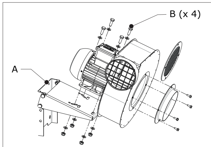
Fig. 4.2 Cómo instalar el ventilador en un MB-FUA-C1/C2
