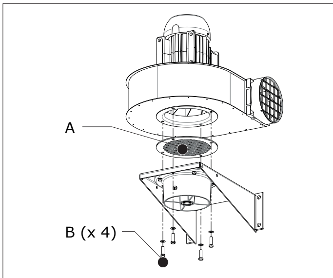
Fig. 4.5 Ventilator direkt an einem Absaugarm montieren
