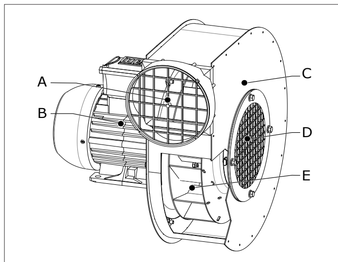
Fig. 2.1 Huvudkomponenter FUA-1300/1800/2100
