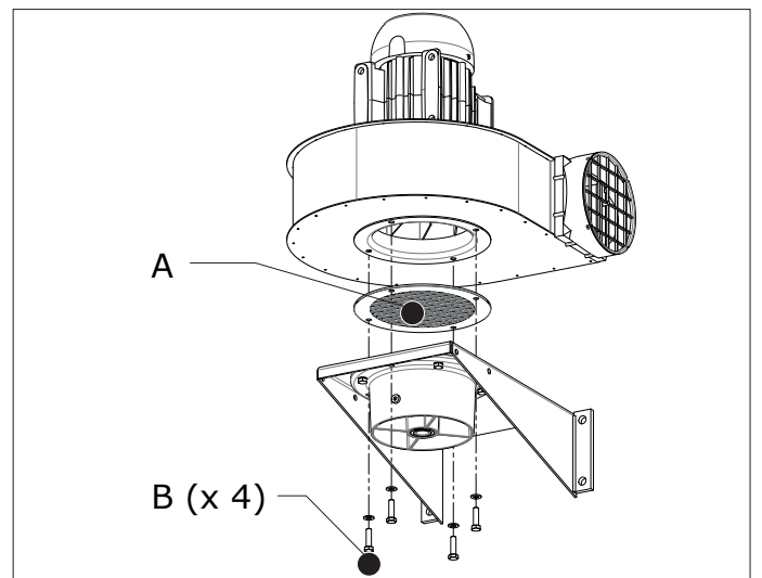
Fig. 4.5 Montering av fläkten direkt på en arm
