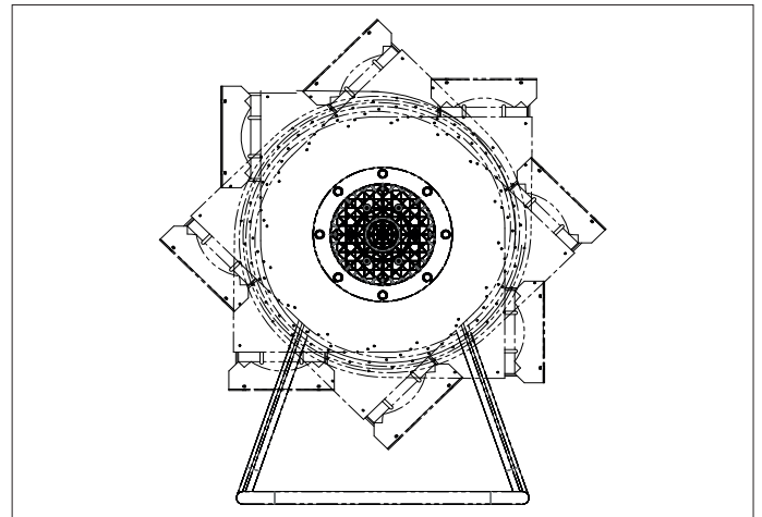
Fig. 4.3 Variabele uitlaatdeelpositie
