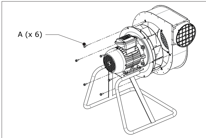
Fig. 4.4 Auslassposition ändern
