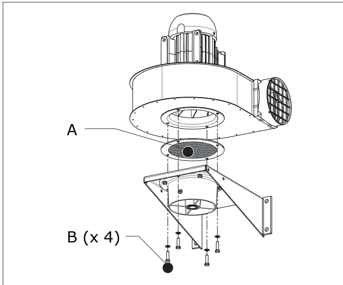
Fig. 4.5 Cómo instalar el ventilador directamente en un brazo
