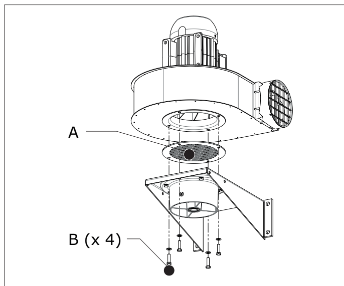
Fig. 4.5 Installation directe du ventilateur sur un bras
