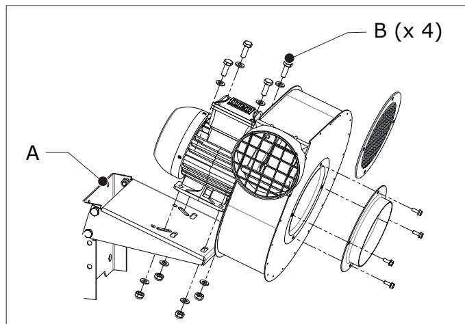
Fig. 4.2 Installation du ventilateur sur un MB-FUA-C1/C2
