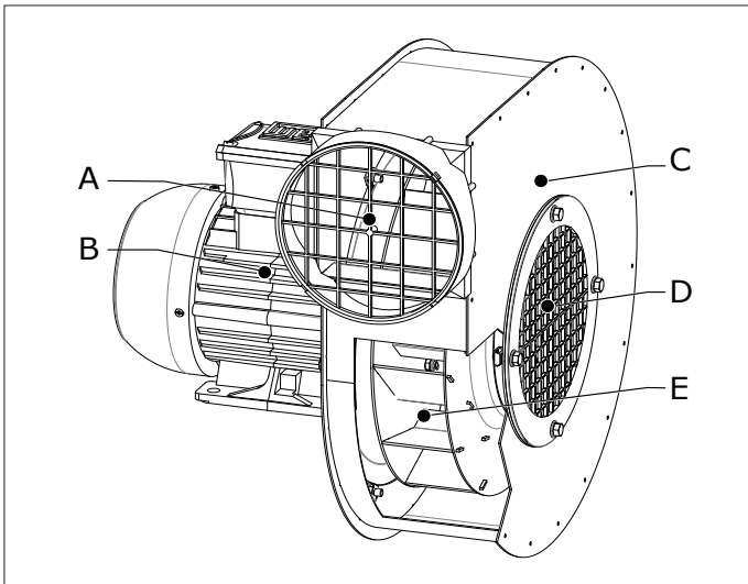
Fig. 2.1 Hoofdcomponenten FUA-1300/1800/2100
