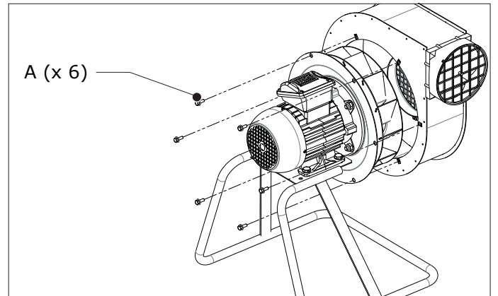
Fig. 4.4 Ändra utloppets riktning
