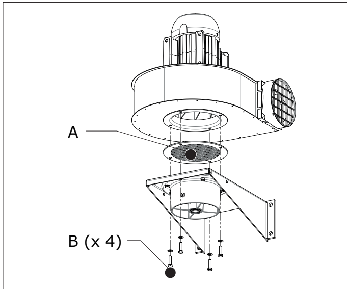
Fig. 4.5 De ventilator rechtstreeks monteren op een arm
