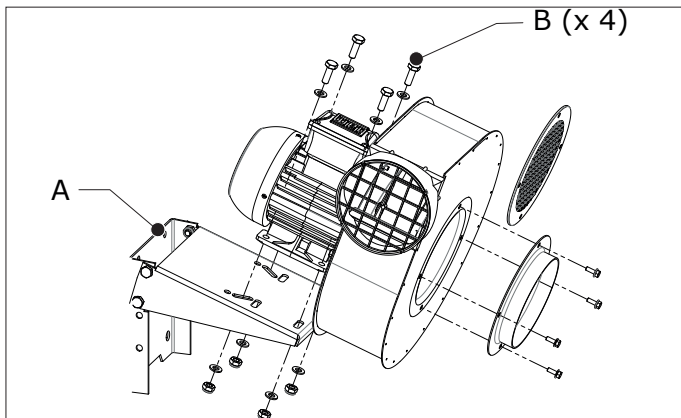
Fig. 4.2 Montering av fläkten på en MB-FUA-C1/C2
