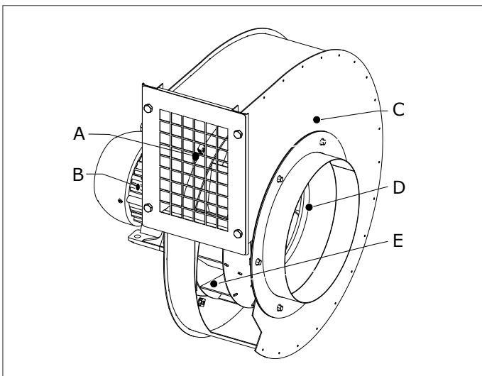
Fig. 2.2 Hoofdcomponenten FUA-3000/4700
