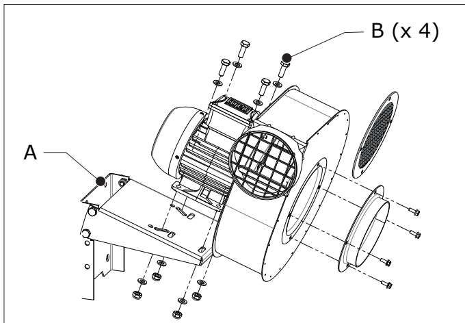
Fig. 4.2 De ventilator monteren op een MB-FUA-C1/C2
