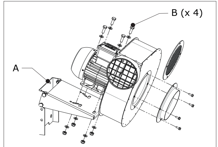
Fig. 4.2 Ventilator an MB-FUA-C1/C2 montieren
