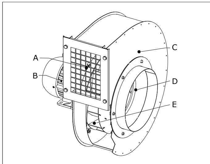
Fig. 2.2 Composants principaux FUA-3000/4700
