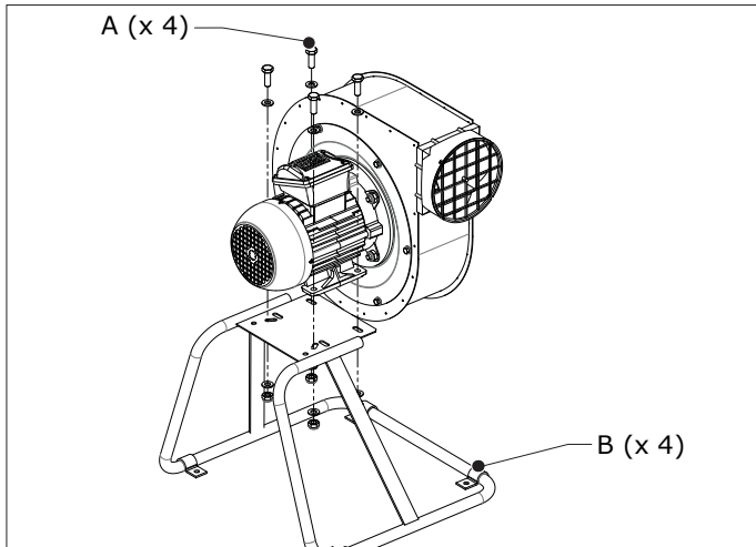
Fig. 4.1 Montering av fläkten på en MB-FUA-S1/S2
