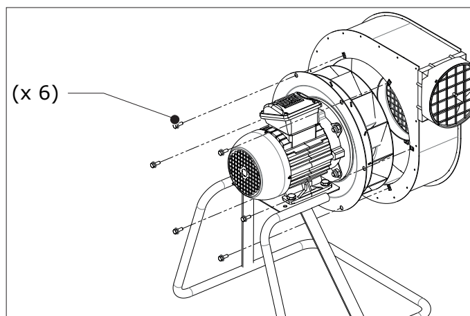
Fig. 4.4 Modification de la position de sortie
