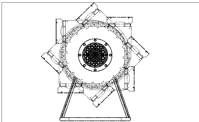
Fig. 4.3 Variabel utloppsposition
