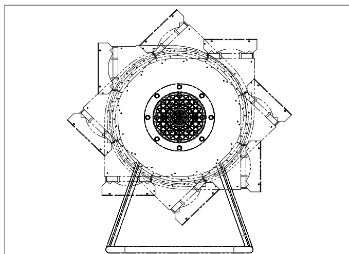
Fig. 4.3 Position d'échappement variable
