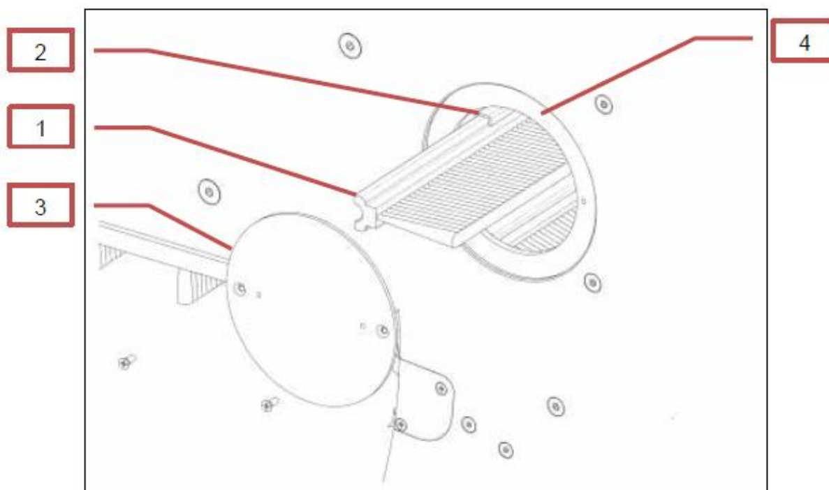
Kuva 1 Harjojen asettaminen
