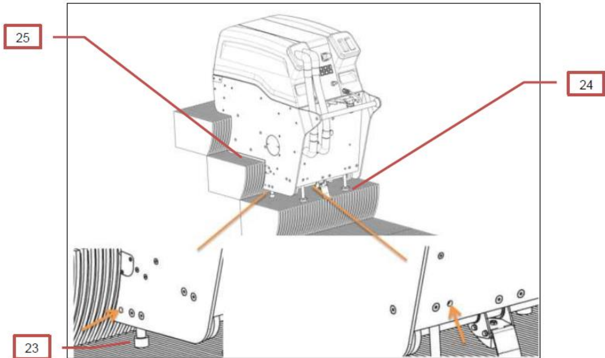
Kuva 5 Porraskorkeuden säätö
