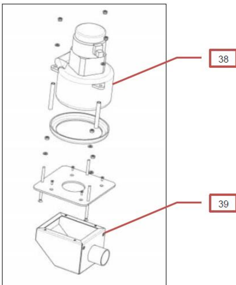
Kuva 20 Keräyssäiliö
