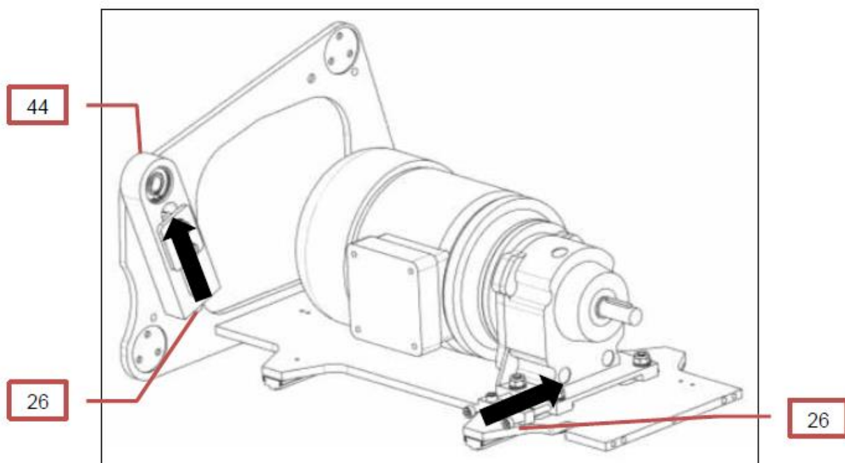
Kuva 23 Ketjujen kiristäminen
