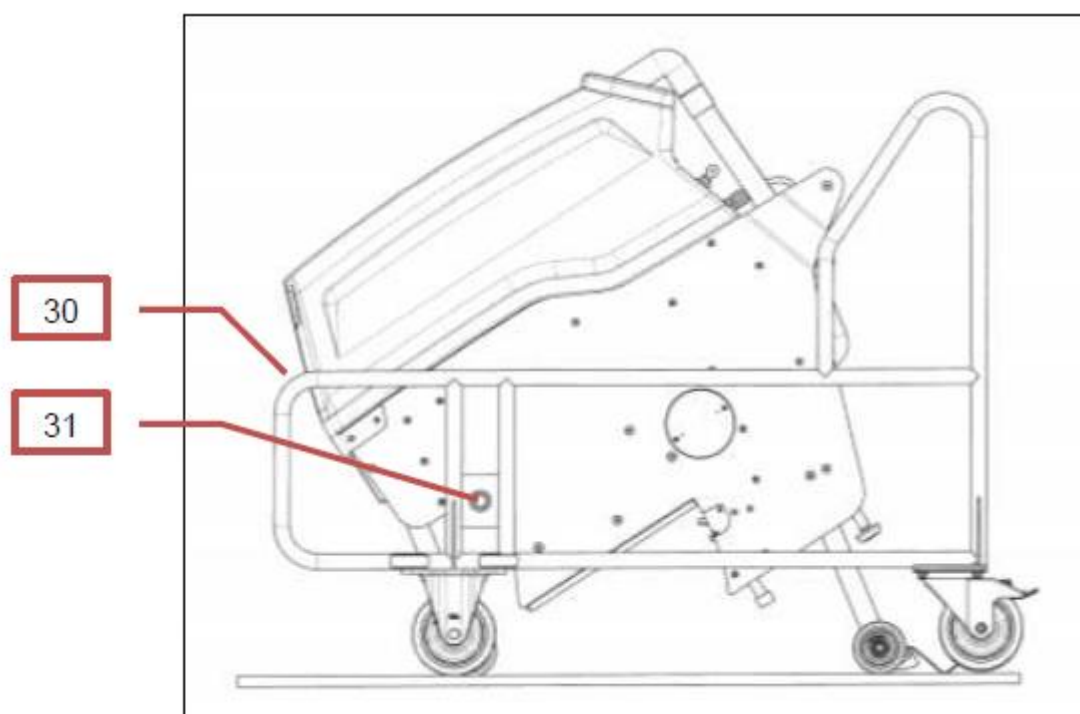
Kuva 15 Siirtäminen kuljetusasentoon
